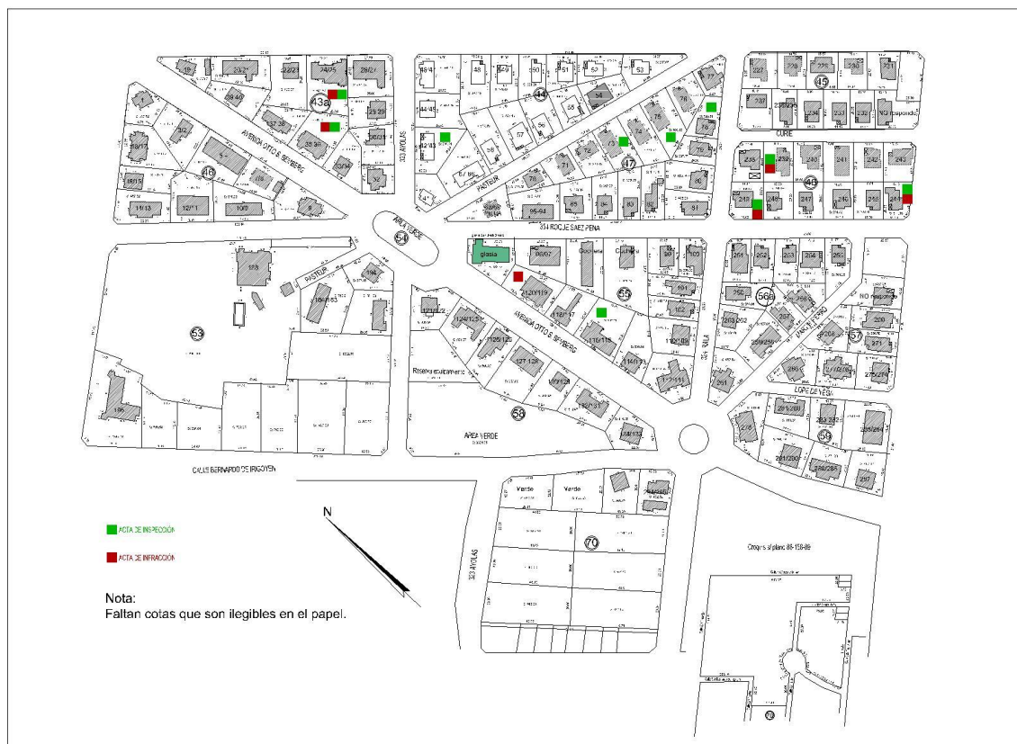
Figura 6. Planimetría general del barrio. Reconstrucción digitalizada.
